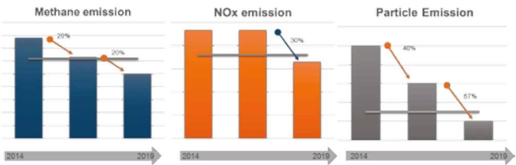
Figuur 2: Ontwikkeling van de Wärtsilä 20 Dual Fuel motor: NRMM Stage V (zonder nabehandeling)
